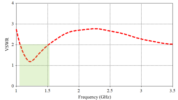
Fig. 9. S-parameter (2 nd antenna).
