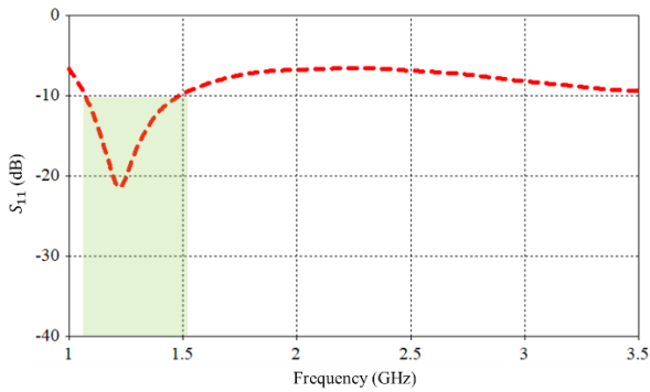
Fig. 5. S-parameter (2 nd antenna).
