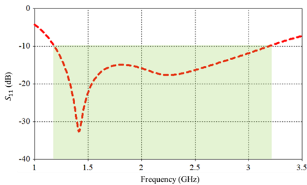
Fig. 2. S-parameter (1 st antenna).
