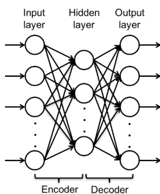
Fig. 6. Autoencoder
