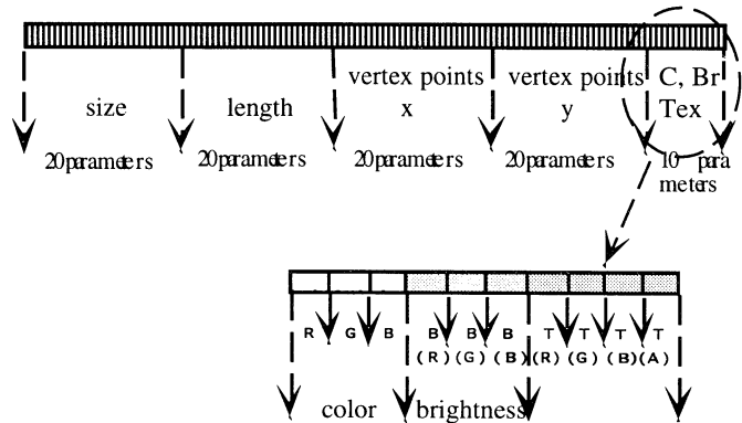
Fig. 3: Genetic String
