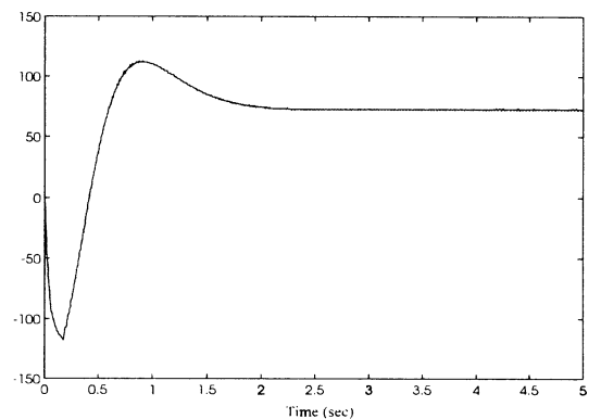
Fig. 4. Actual Control Signal \tau
