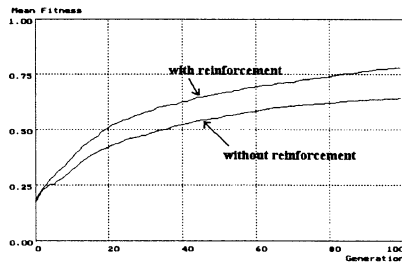
Fig. 3 Population : 100
