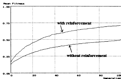
Fig. 4 Population : 50
